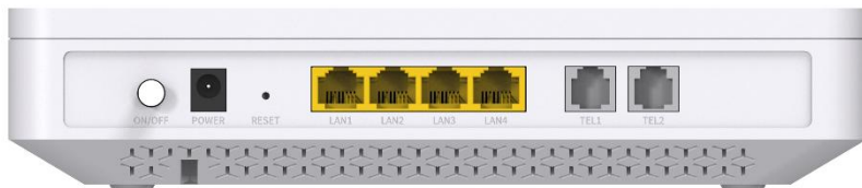
Rys. 2 Panel tylny
